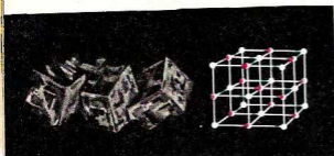
Chlorek sodu (sól kuchenna — NaCl)
